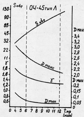
Рис. 2. Кривые зависимости светочувствительности S_{0\text{пр}} , коэффициента контрастности \gamma , максимальной оптической плотности D_{\text{макс}} и минимальной оптической плотности D_{\text{мин}} от времени первого проявления t_{\text{пр}} плёнки ОЧ-45 типа Л.
