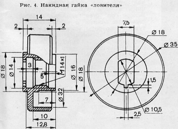
Рис. 4. Накидная гайка «ловителя»
